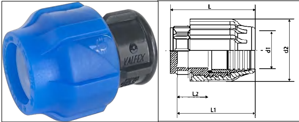
Рисунок 10. Заглушка компрессионная
