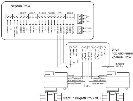
Рис. 2 Схема подключения кранов серии Neptun Bugatti Pro 220 В к блоку подключения кранов и подсоединения блока подключения кранов ProW к модулю управления Neptun ProW.
