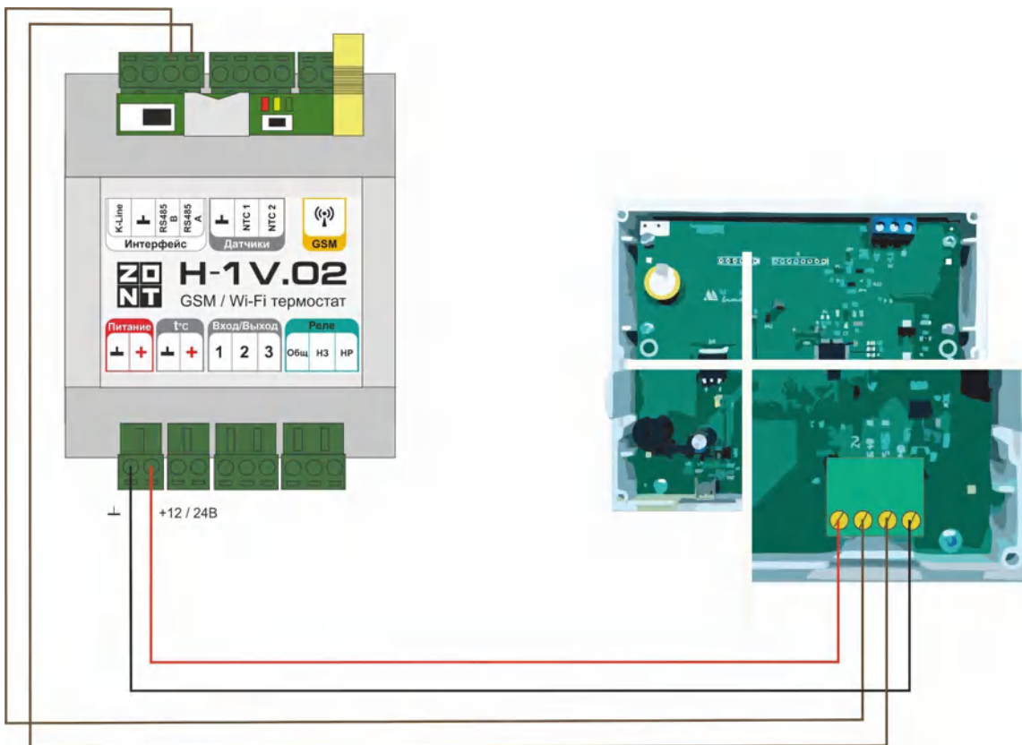
Пример подключения 3-х панелей по интерфейсу RS-485 :
