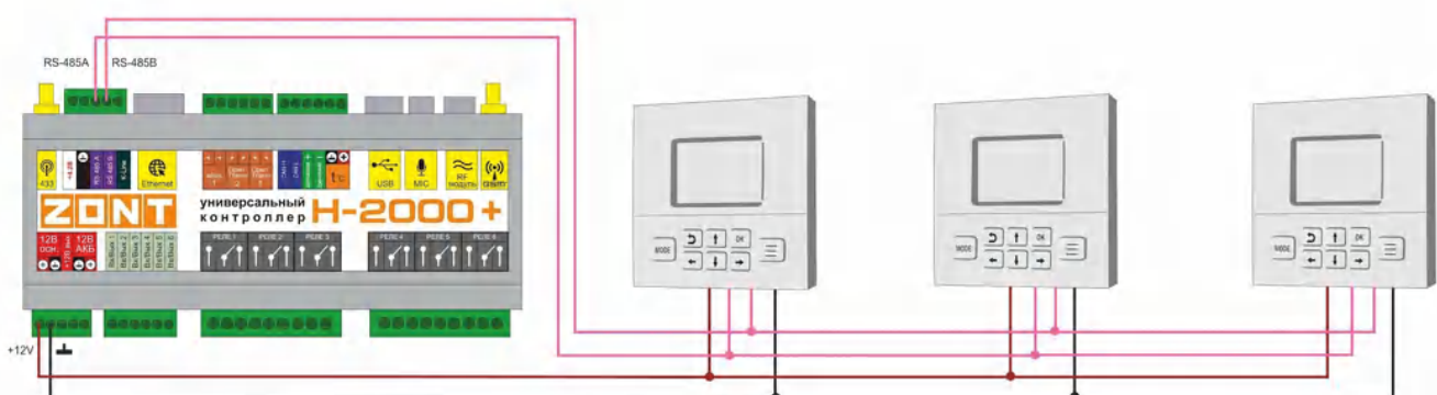
Пример подключения 3-х панелей по интерфейсу RS-485:
