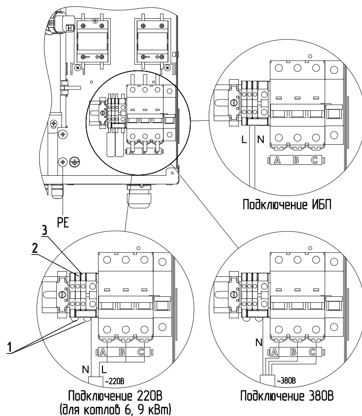
Рис.7 Схема подключения электрического котла ZOTA SOLID-X 6-24 кВт
