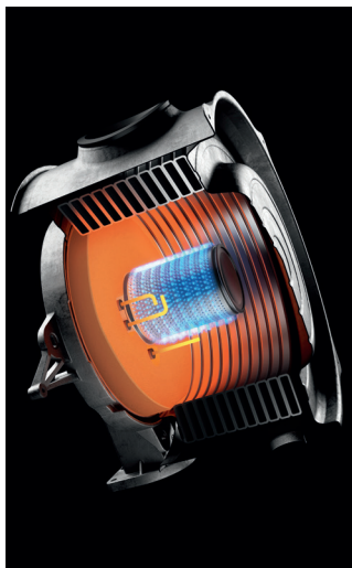
Горелка MatriX-Plus
